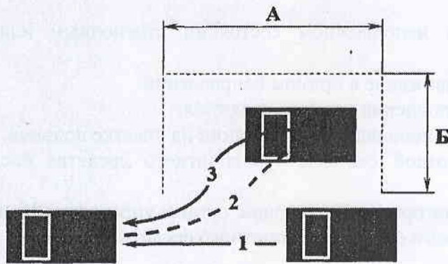
Рисунок 4. Схема и размеры маневра "Постановка транспортного средства на место стоянки параллельно тротуару (краю проезжей части) при движении задним ходом"
