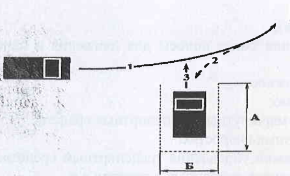
Рисунок 2. Схема и размеры маневра "Постановка транспортного средства на место стоянки при движении задним ходом с поворотом на 90 градусов"
