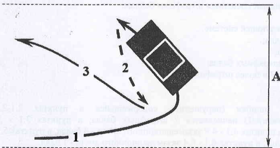
Рисунок 5. Схема маневра "Разворот транспортного средства в ограниченном пространстве (при ограниченной ширине проезжей части) с использованием движения задним ходом"
